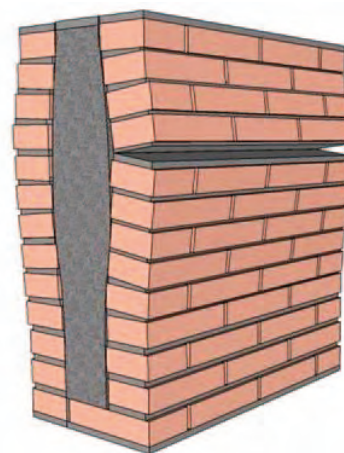
Figura 10: modalità di rottura tipica delle murature multi-paramento con nucleo incoerente: una delle due cortine viene interessata da fenomeni di instabilità che provoca il collasso del pannello.
