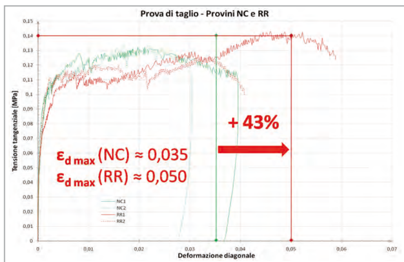
Figura 15: confronto dei grafici tensione tangenziale/deformazione diagonale dei provini di muratura “a sacco” sottoposti a prova di taglio. Nei provini rinforzati con TICORAPSIMO “RR” (curve in rosso) si nota rispetto al caso “non consolidato” (curve in verde), un aumento degli spostamenti ed un’incremento della pseudo-duttilità.
