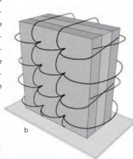
Figura 7: le due diverse disposizioni del rinforzo applicate nei provini testati in laboratorio: localizzato solo nei giunti di malta orizzontali “RO” (a) o sia nei giunti orizzontali che verticali, disposizione denominata “a reticolo”, “RR” (b).
