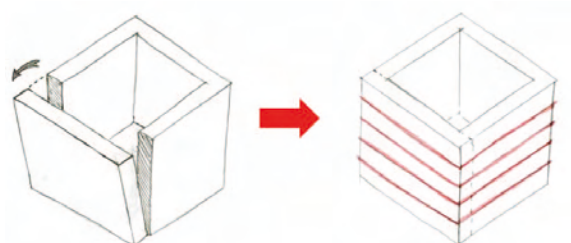
Figura 5: TICORAPSIMO® è ideale anche per una eventuale messa in sicurezza in casi di emergenza
