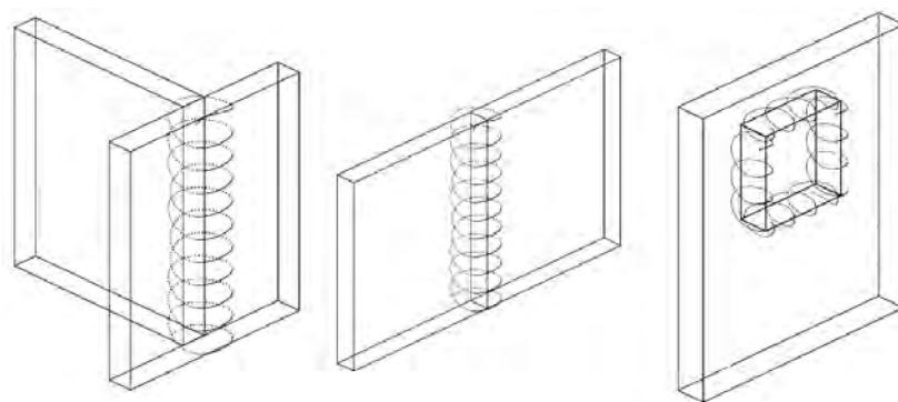
Figura 4: TICORAPSIMO® può essere utilizzato anche per ripristinare la continuità della muratura in presenza di lesioni o carenza di ammassamento e per migliorare le connessioni strutturali tra murature e solai e coperture
