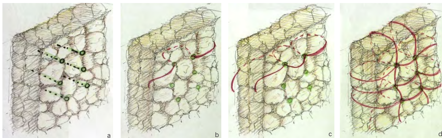
Figura 3: le fasi dell'intervento con TICORAPSIMO®: esecuzione di fori passanti (a), inserimento della corda in fibra di basalto (b) in modo da creare una "maglia" con funzione di collegamento e contenimento degli elementi costituenti la muratura (c, d).
