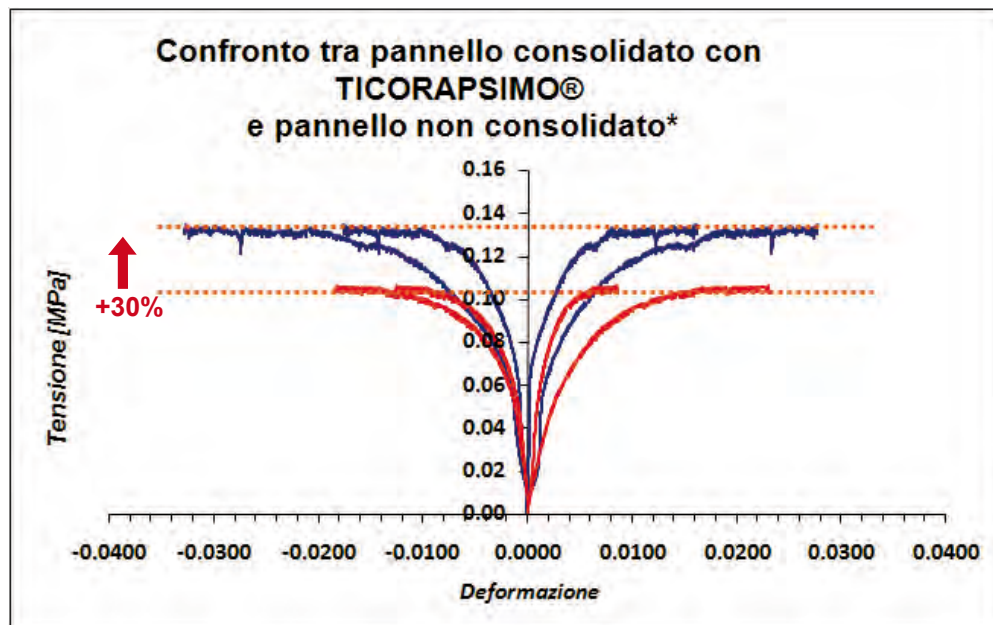
Figura 20: Confronto tra pannello rinforzato con TICORAPSIMO® e pannello non rinforzato sottoposti a prova di compressione diagonale confinata secondo le condizioni in situ
