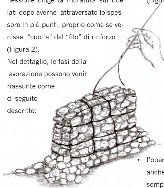
Figura 2: L'idea delle cuciture per consolidare la muratura: il sistema TICORAPSIMO®. In pratica, un elemento continuo e flessibile cinge la muratura sui due lati dopo averne attraversato lo spessore in più punti, proprio come se venisse, appunto, "cucita" dal "filo" di rinforzo.
