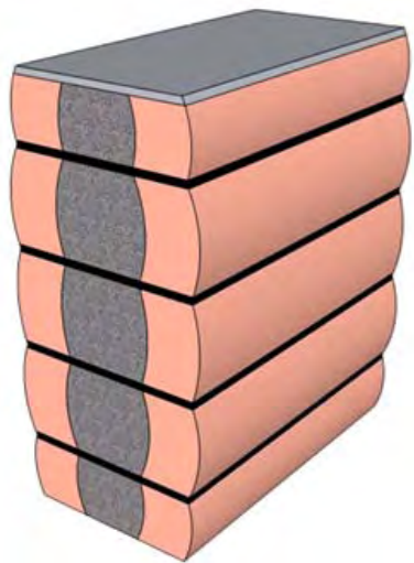
Figura 1: l'applicazione di TICORAPSIMO® fornisce monoliticità al pannello murario: si modifica la modalità di rottura, scongiurando rotture per instabilità delle cortine esterne, consentendo di sfruttare al meglio i materiali costituenti la muratura.
