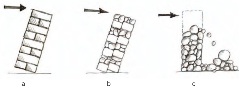
Figura 1: Risposta della muratura ad azioni orizzontali fuori dal piano: se è di “buona qualità” (a) ci si può aspettare un comportamento monolitico, al contrario, se è di “scarsa qualità” (b) si disgrega caoticamente. In caso di “media qualità” dell’apparecchio murario (c), ci si deve aspettare un comportamento intermedio. L’attivazione di meccanismi di collasso in caso di sisma è subordinata alla capacità della muratura di comportarsi in maniera monolitica.
