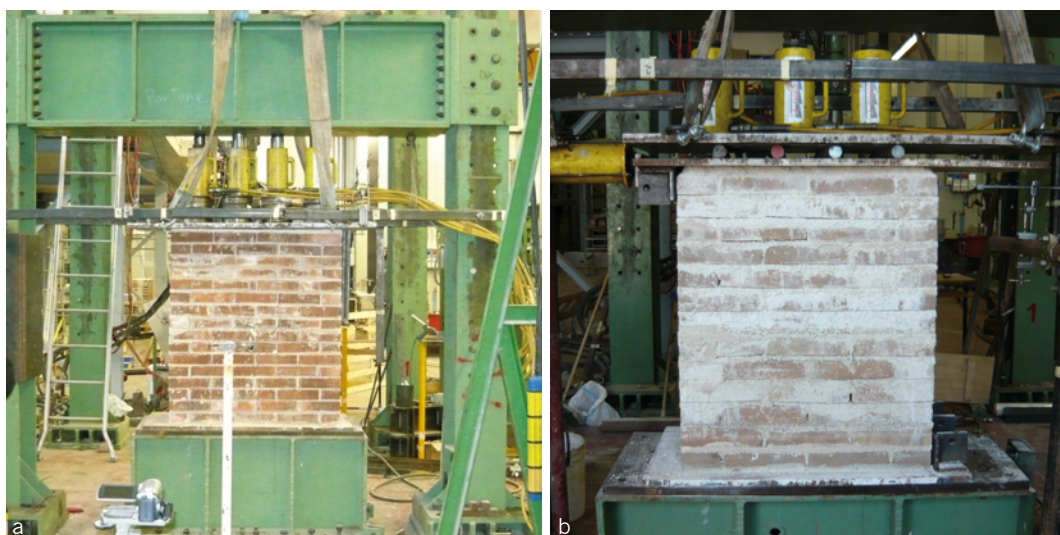
Figura 9: dispositivi di prova allestiti in laboratorio per l'esecuzione di prove di compressione verticale (a) e di prove a taglio (b).
