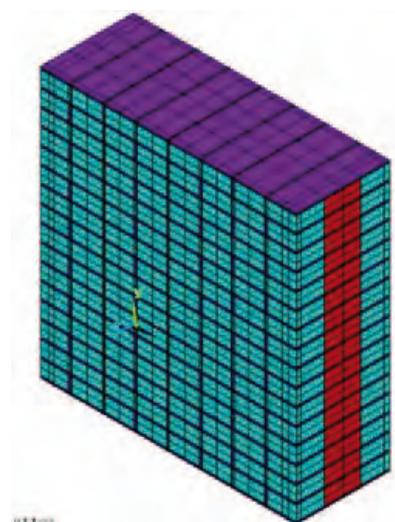
Figura 17: modello FEM utilizzato per riprodurre le prove sperimentali eseguite in laboratorio.
